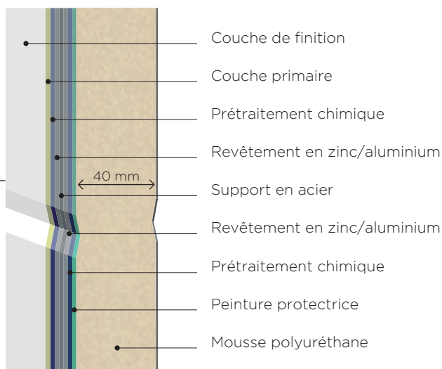
Coupe d'un panneau
