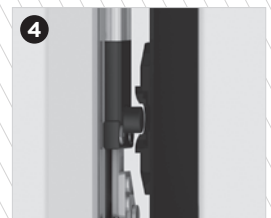
Gâches de centrage du portillon en position fermée
