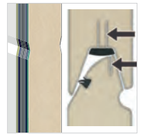
Remplissage panneaux acier à RPT (1) et mousse isolante 40 mm
