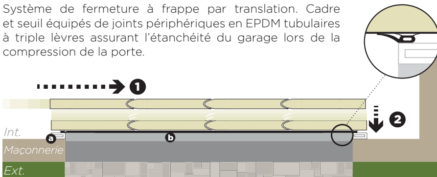
a Cadre b Seuil + joint Exemple pour une porte de garage en 4 panneaux vue du dessus
