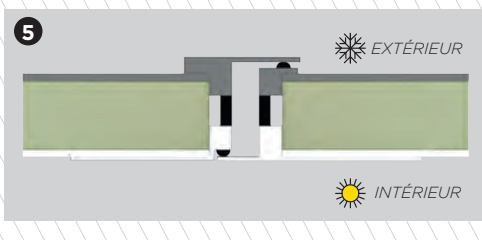
Profils à rupture de pont thermique
