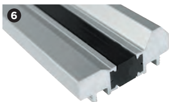
Seuil en aluminium à rupture de pont thermique (hauteur : 20 mm)
